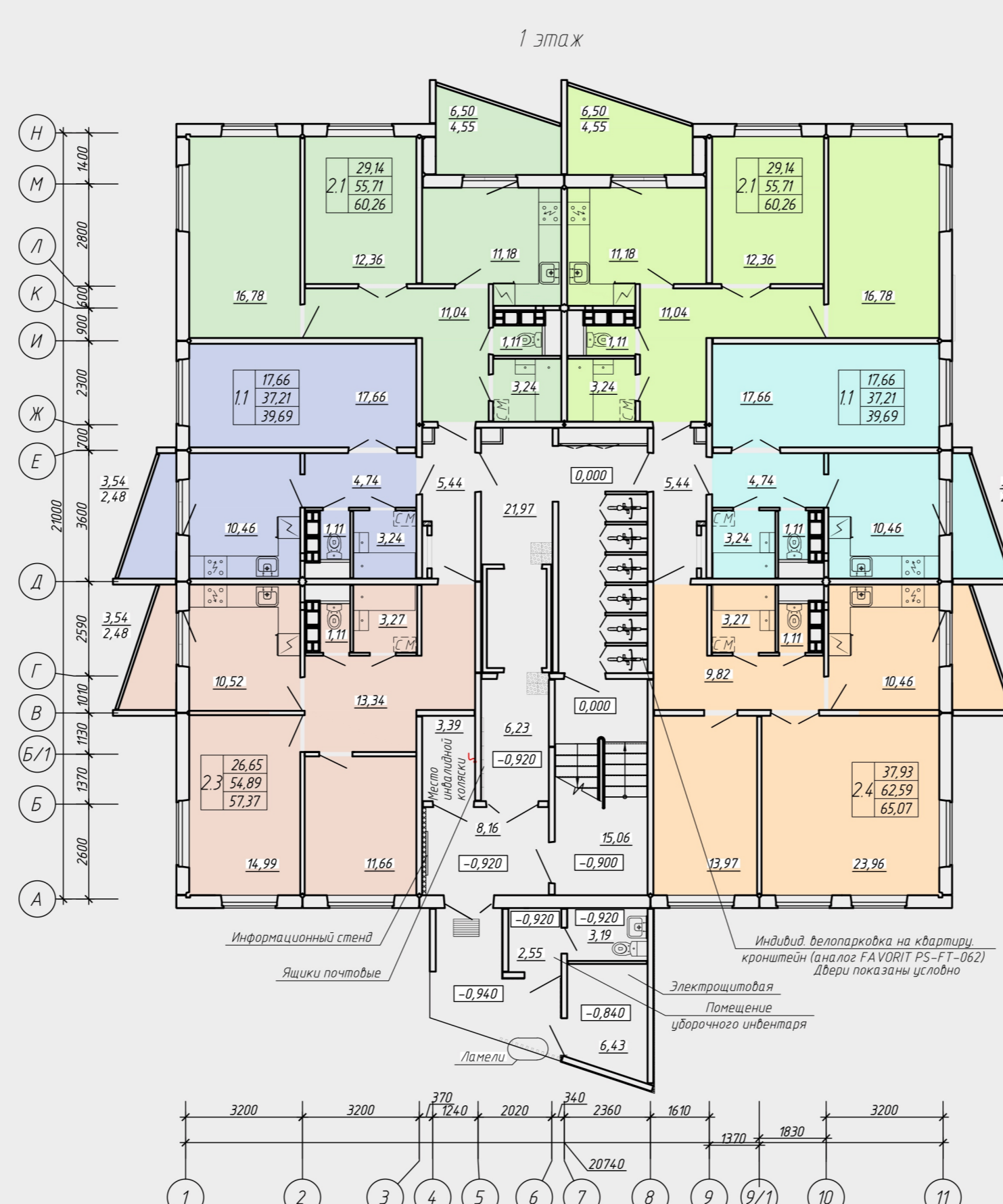
План первого этажа
