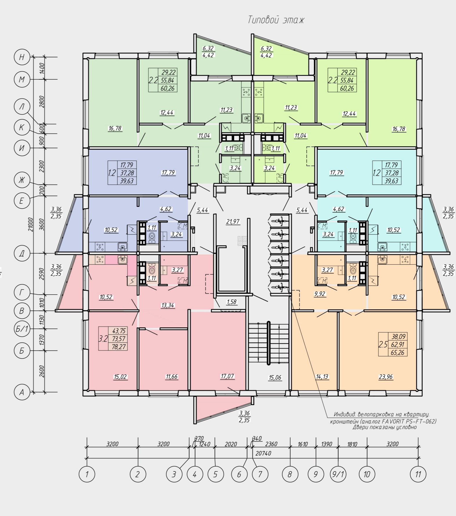
План типового этажа
